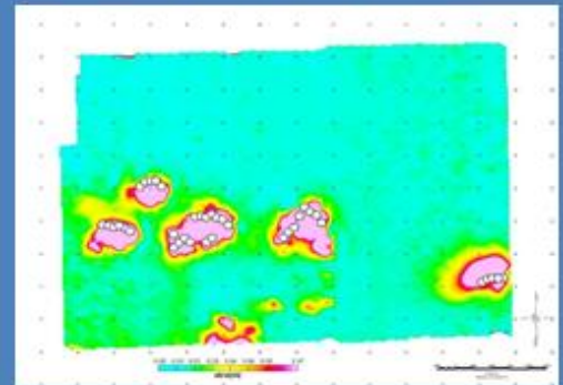
DEEP RESPONSE EM CONDUCTORS
